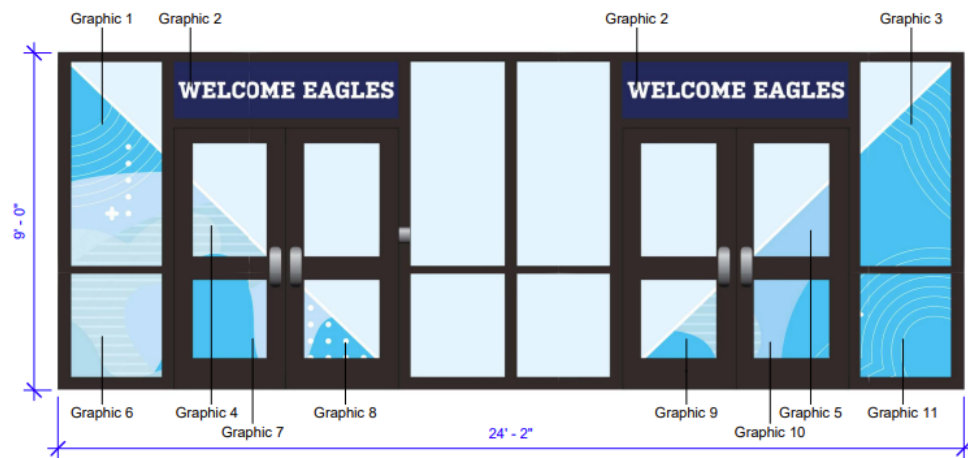
① Elevation 1 1 : 35
