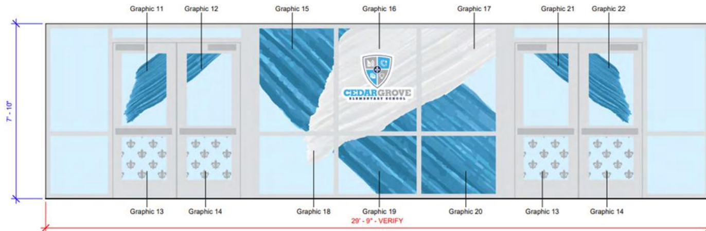
① Elevation 1 1 : 28
