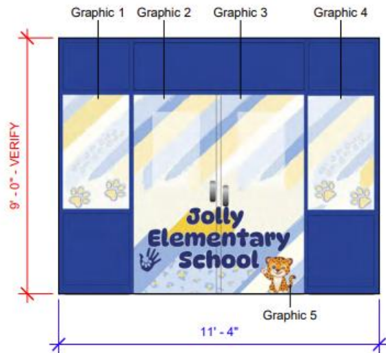
① Elevation 1 1 : 40
