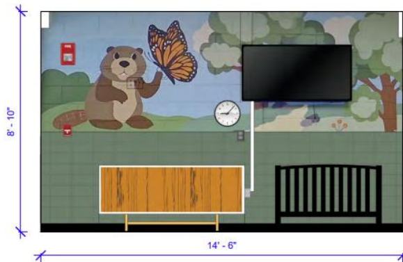
④ Elevation 4 1 : 35
