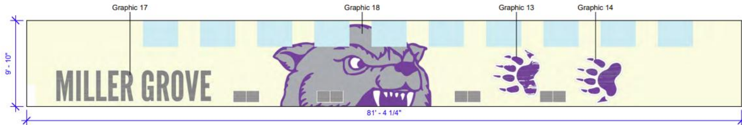
⑨ Elevation 9 1 : 75
