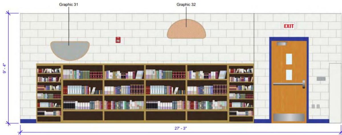
④ Elevation 4 1 : 30
