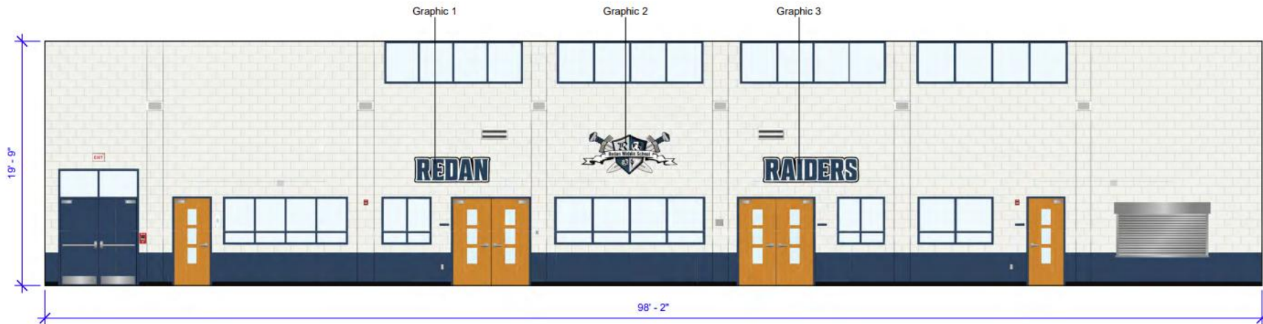
① Elevation 1 1 : 75
