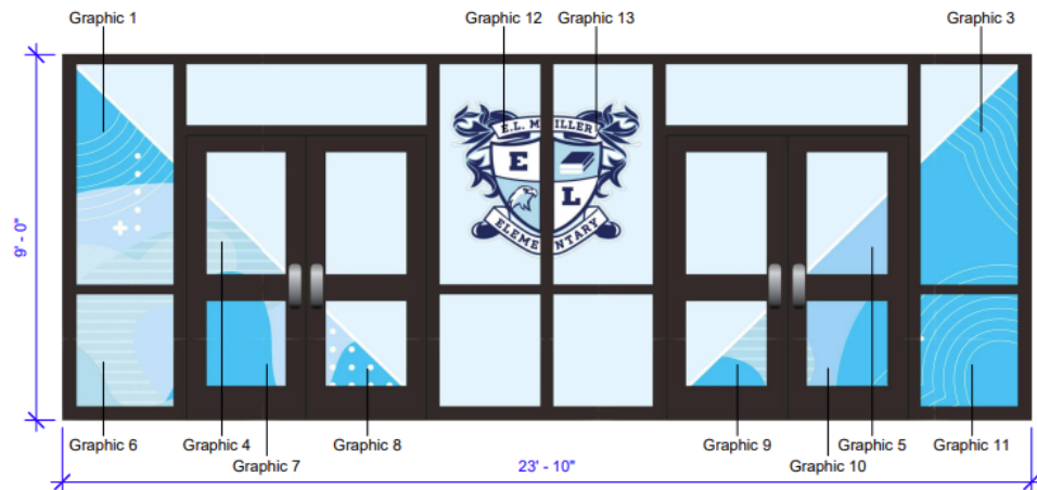
② Elevation 2 1 : 35
